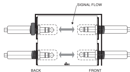
(D) De-Normalled Patchbay
