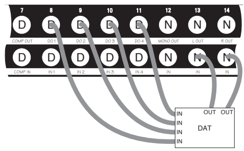
(D) Patching a Multitrack Tape Recorder Into The System
